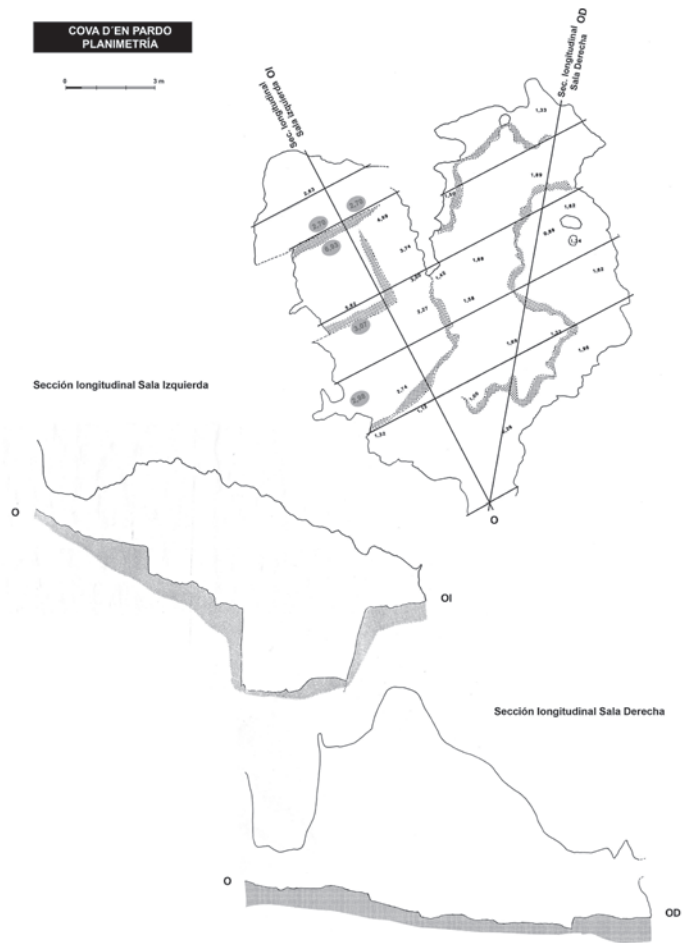
Figura 3.17. Cotas de la cavidad tras los trabajos de limpieza de 1993 y 1996. Destacan la cotas seleccionadas para la reconstrucción de las iniciales de la excavación de 1965.
