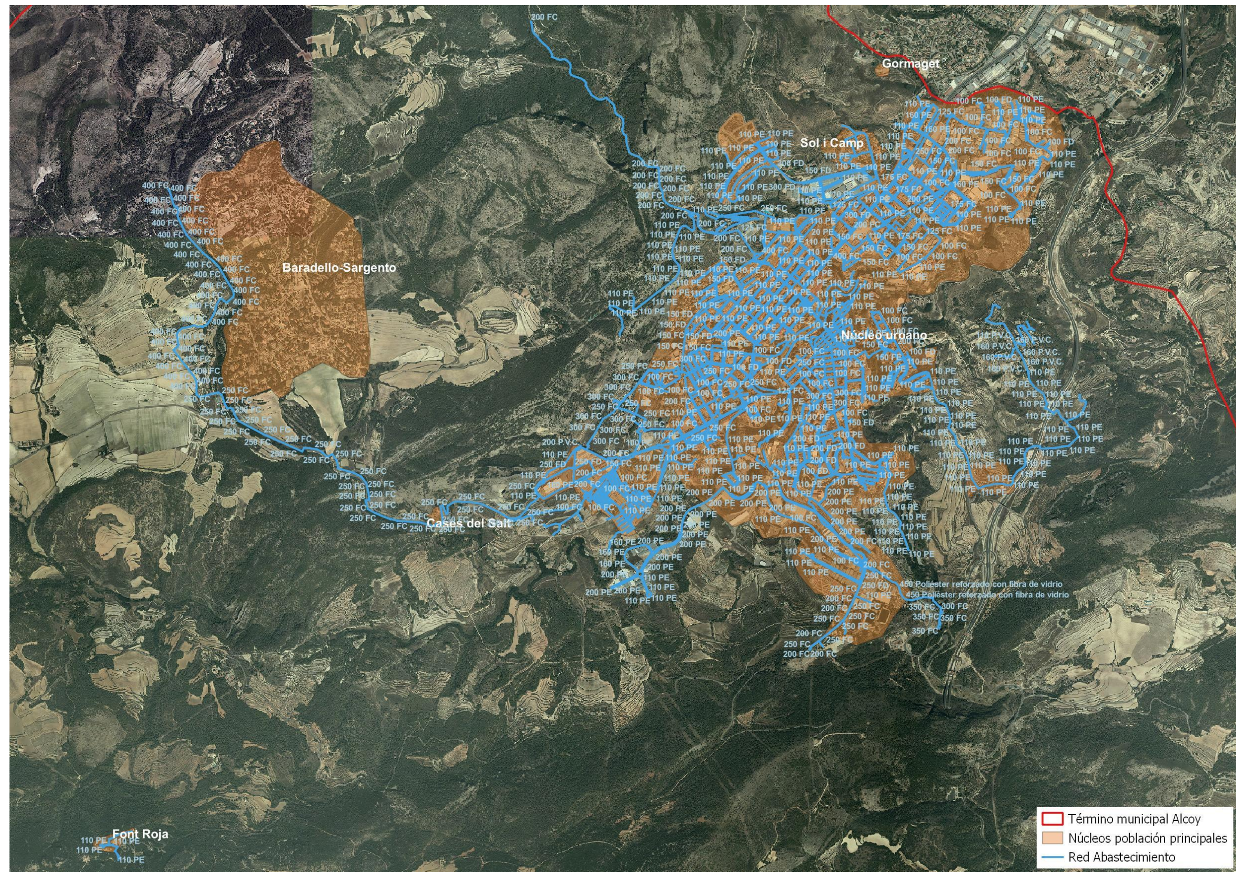
Figura 115.Red municipal de abastecimiento de agua potable de Alcoi
