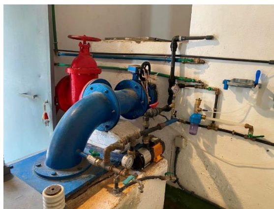
Figura 25. Tubería de impulsión
