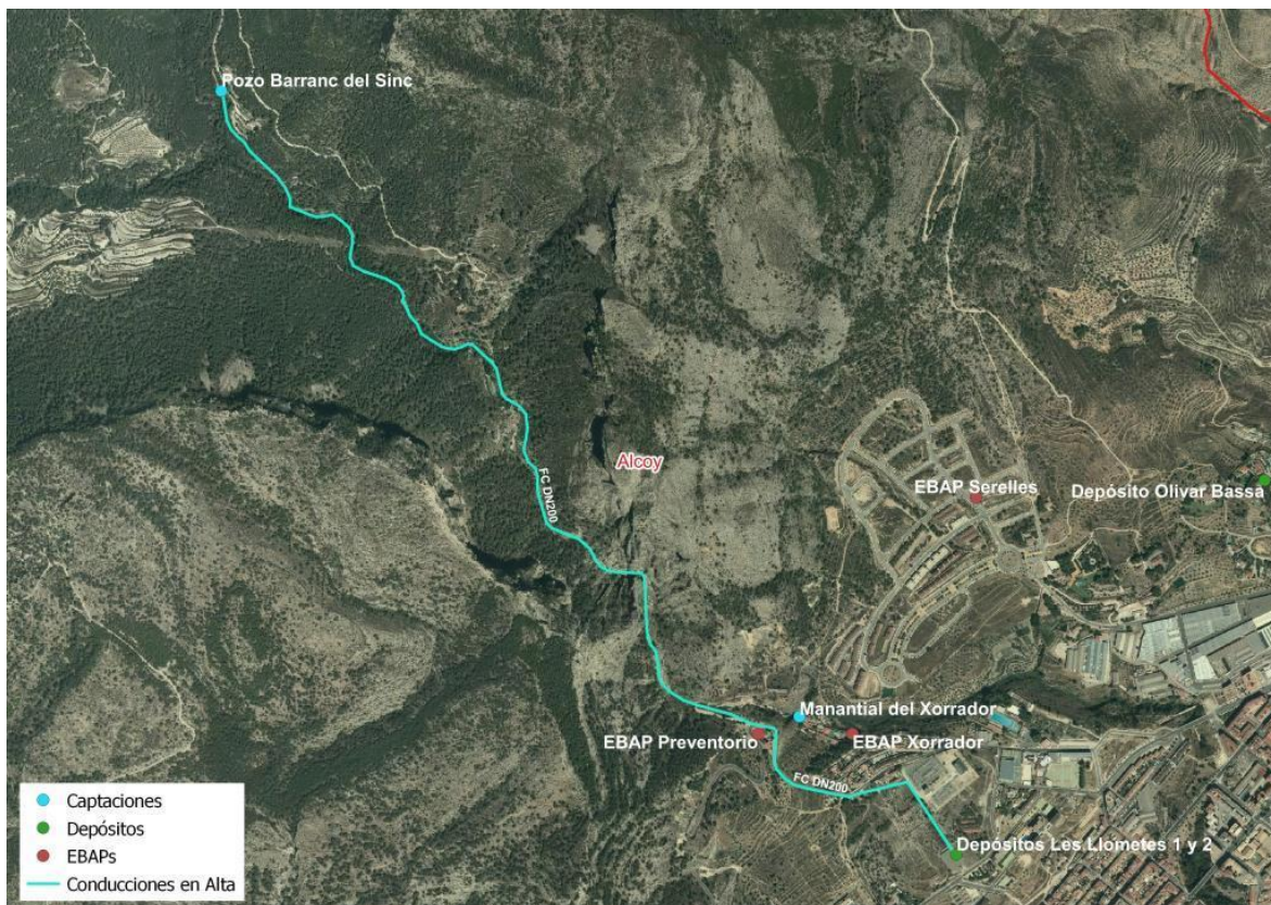
Figura 111. Conducción Pozo Barranc del Sinc-Depósitos Llometes
